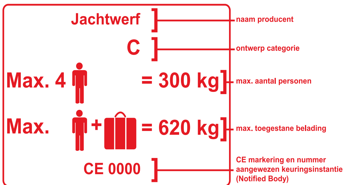
Voorbeeld bouwersplaatje
